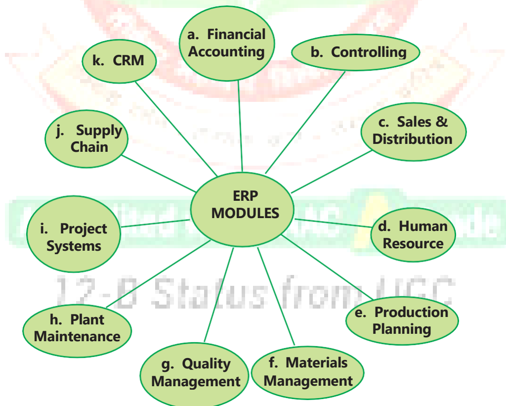
Fig. 2.6.3: ERP Modules
