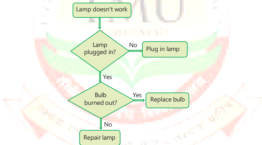
Fig. 1.7.2: Simple Flowchart
